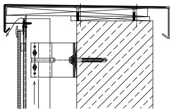
Attikafedéshez csatlakozás
