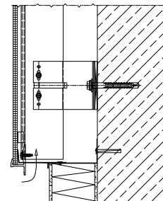
Lábazati csatlakozás
